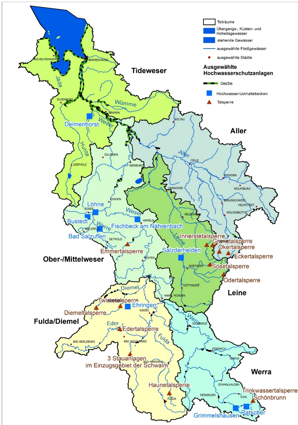
Abb. 5-10: Ausgewählte Hochwasserschutzanlagen in der Flussgebietseinheit Weser (Stand: 19.03.2020 aus FGG WESER 2020a)
